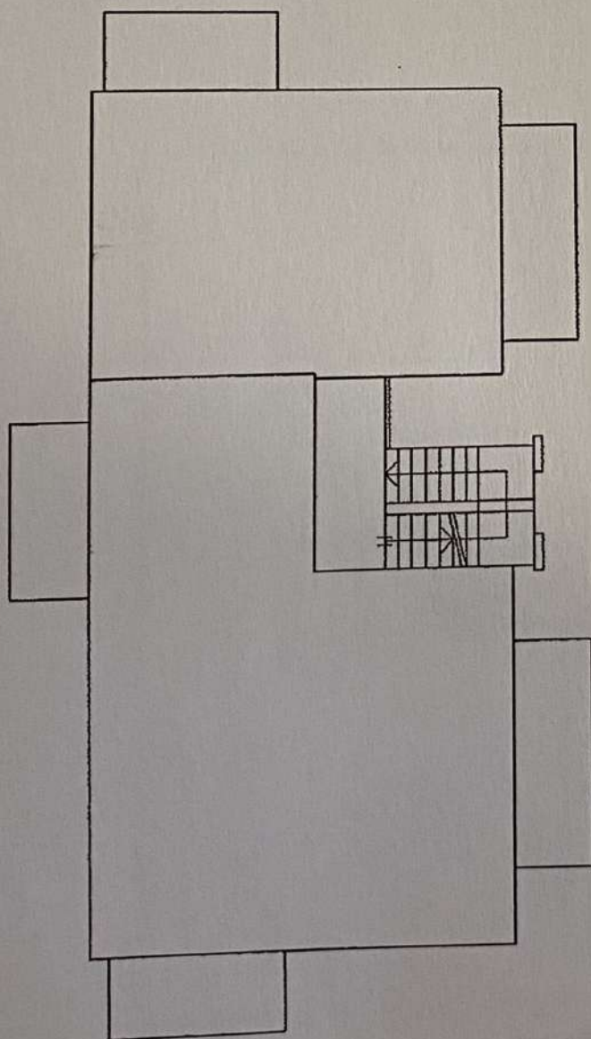
PIANO PRIMO H=2.70
